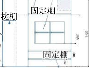
DOMA スペース詳細図
